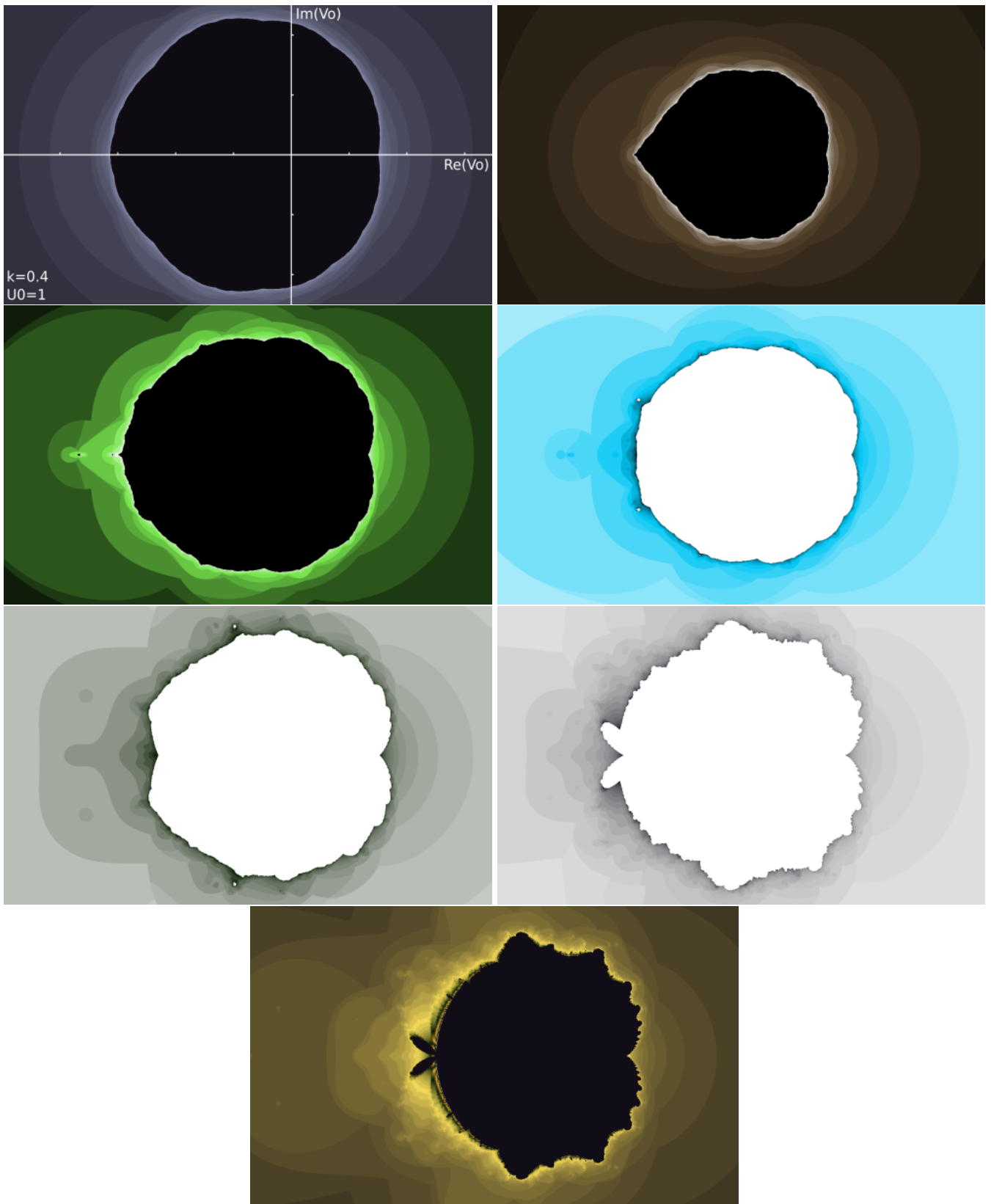
FIG. 4 – Projection de Béryl sur le plan u_0 = 1 , pour k valant successivement 0.4, 0.6, 0.7, 0.75, 0.9, 0.99 et 1
